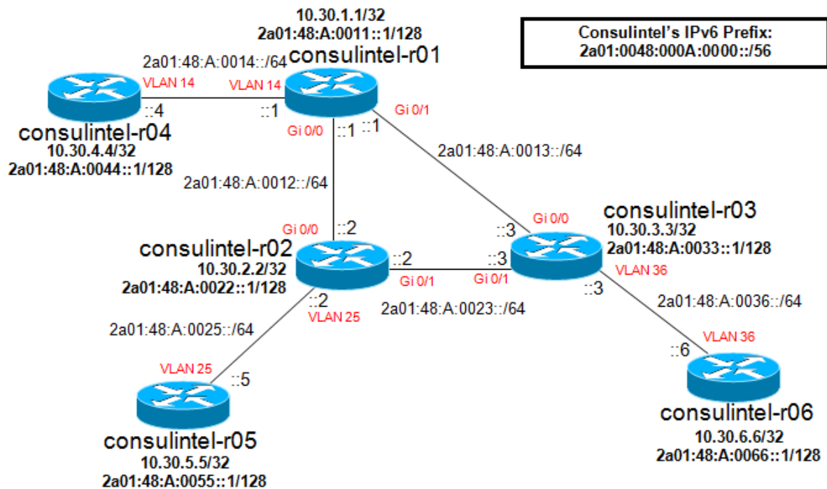
Esquema Testbed Madrid
